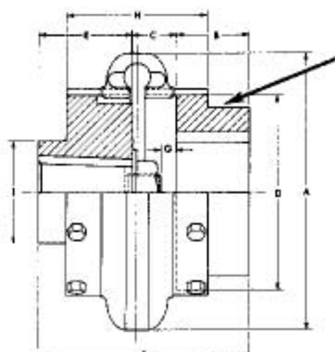
Dimensiones de los acoplamientos para motor de molino
