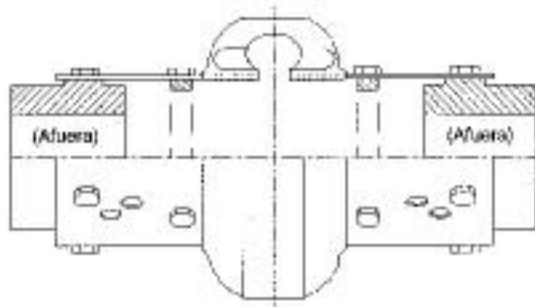
Figura A Ambas mazas montadas hacia afuera
