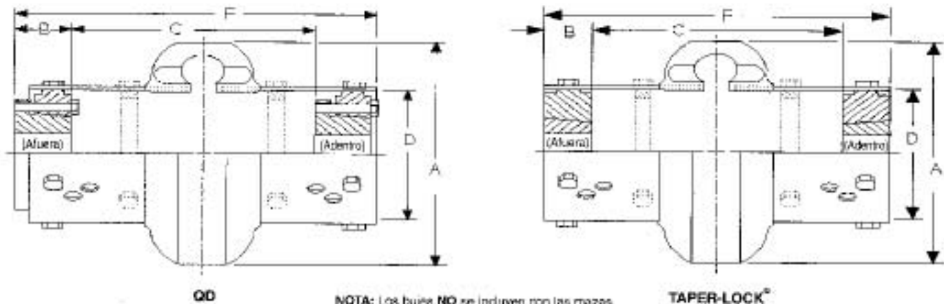
Especificaciones con mazas QD
