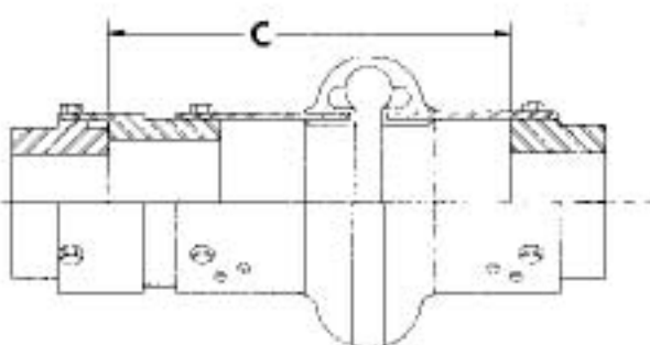
Mazas con barreno recto con extensión sencilla
