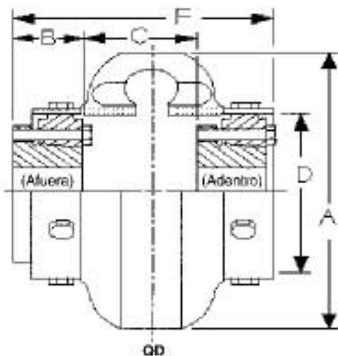
Especificaciones con mazas QD
