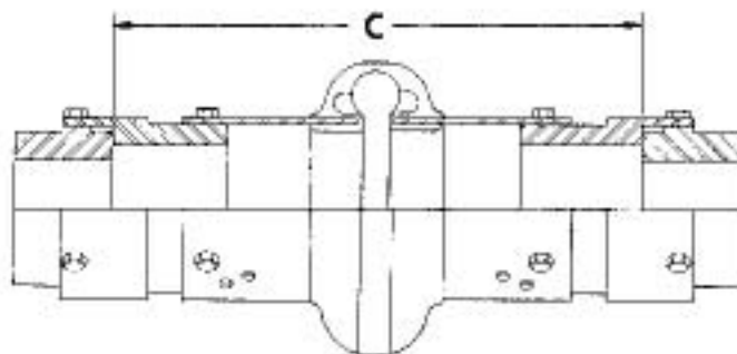
Mazas con barreno recto con doble extensión
