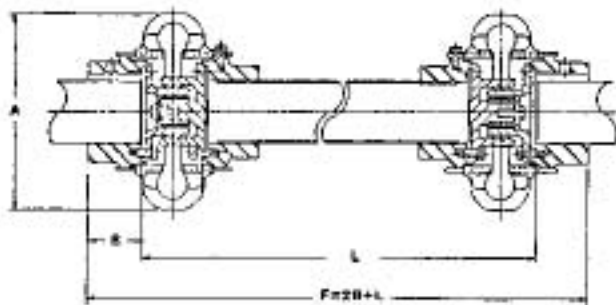
Ensamblaje Tubular Flotante (FTA)
