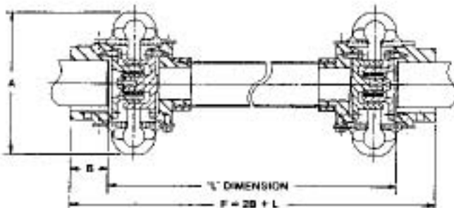
Ensamblaje Tubular Flotante Compuesto Omega (CFTA)
