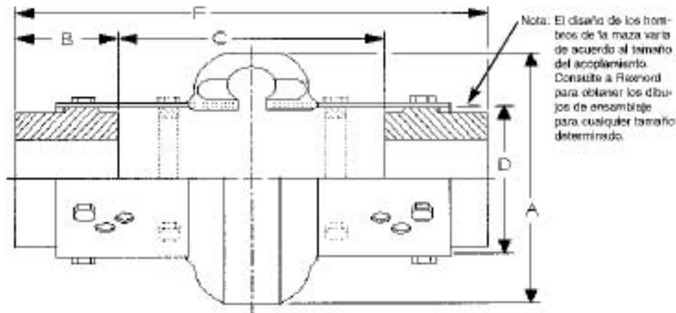
Especificaciones para mazas de barrenado recto
