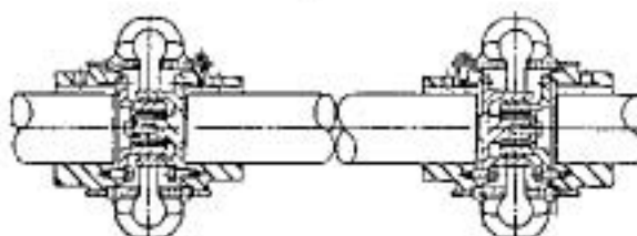
Ensamblaje con eje flotante (FSA)
