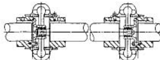
Ensamblaje con eje piloteado (PSA)
