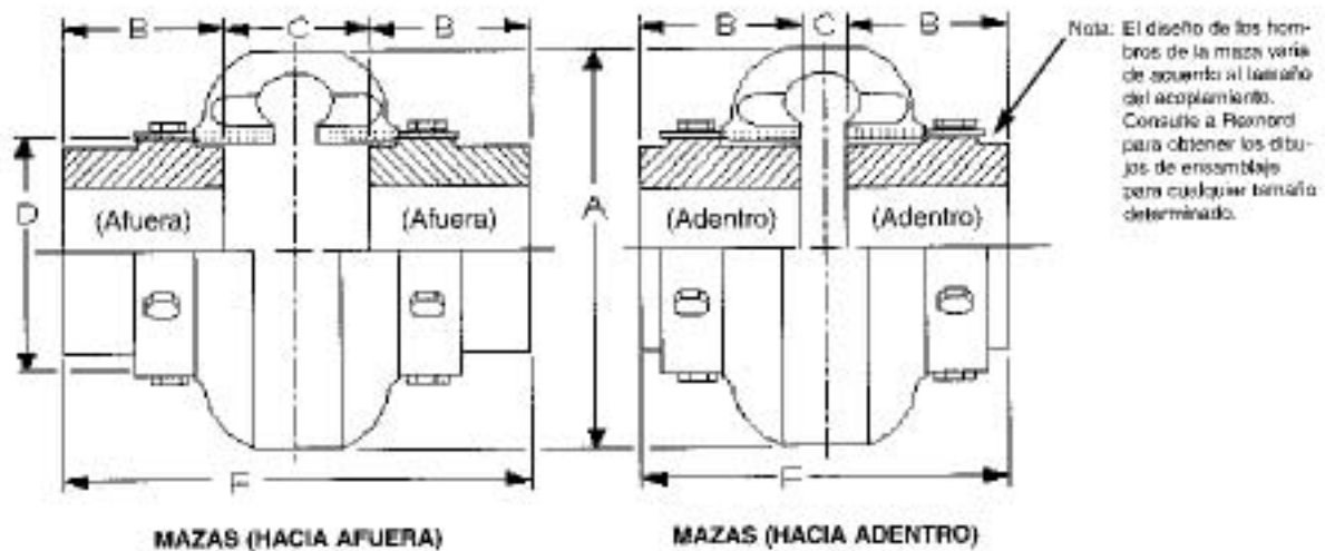
Especificaciones para mazas con barrenado recto
